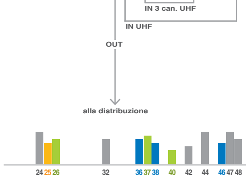
Canali UHF amplificati all'uscita del centralino
